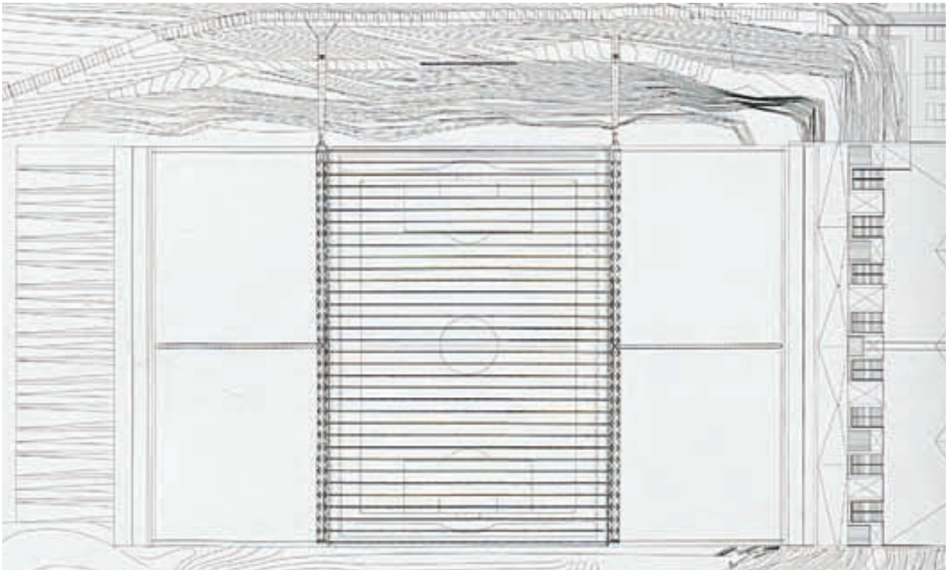
plan de toiture
