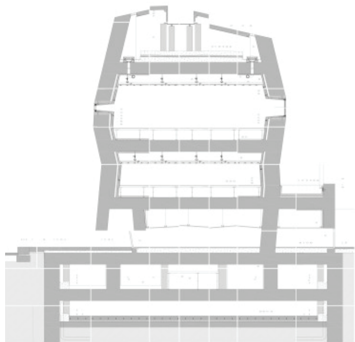
coupe transversale
