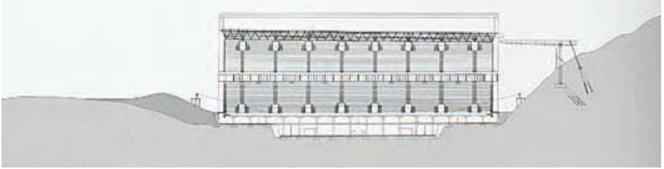
élévation Nord
