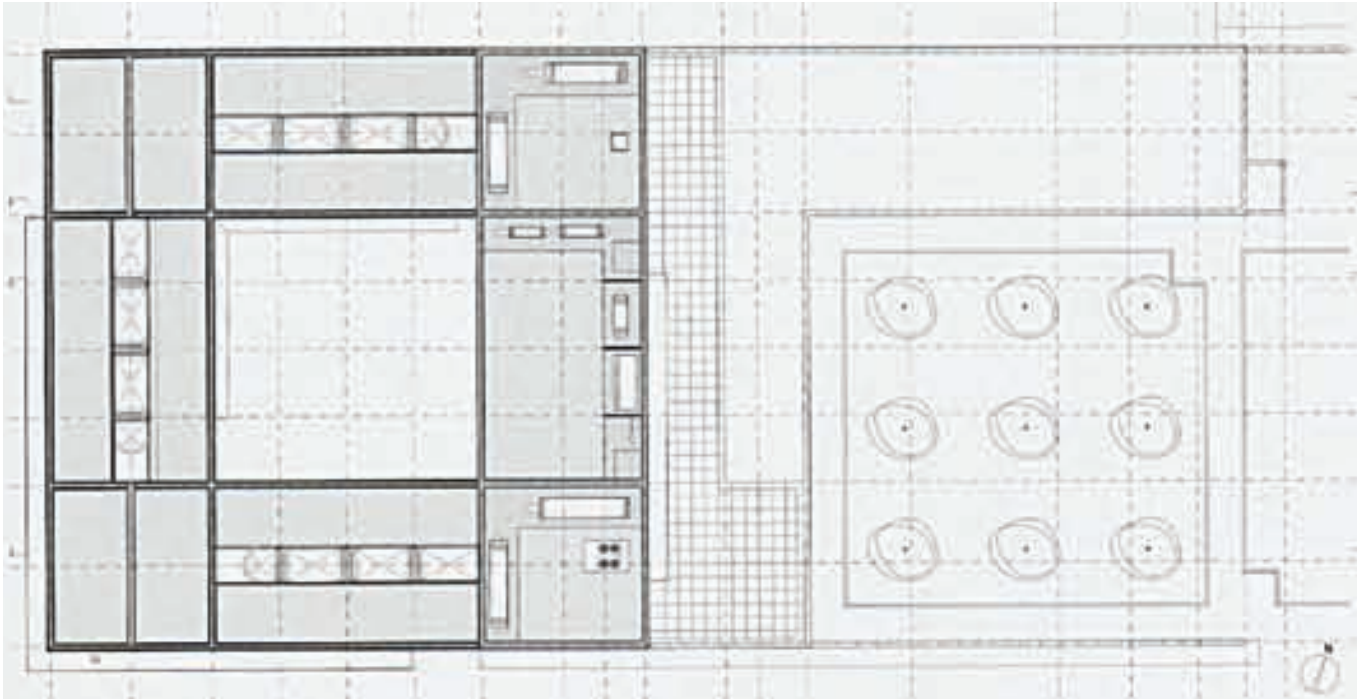
plan attique
