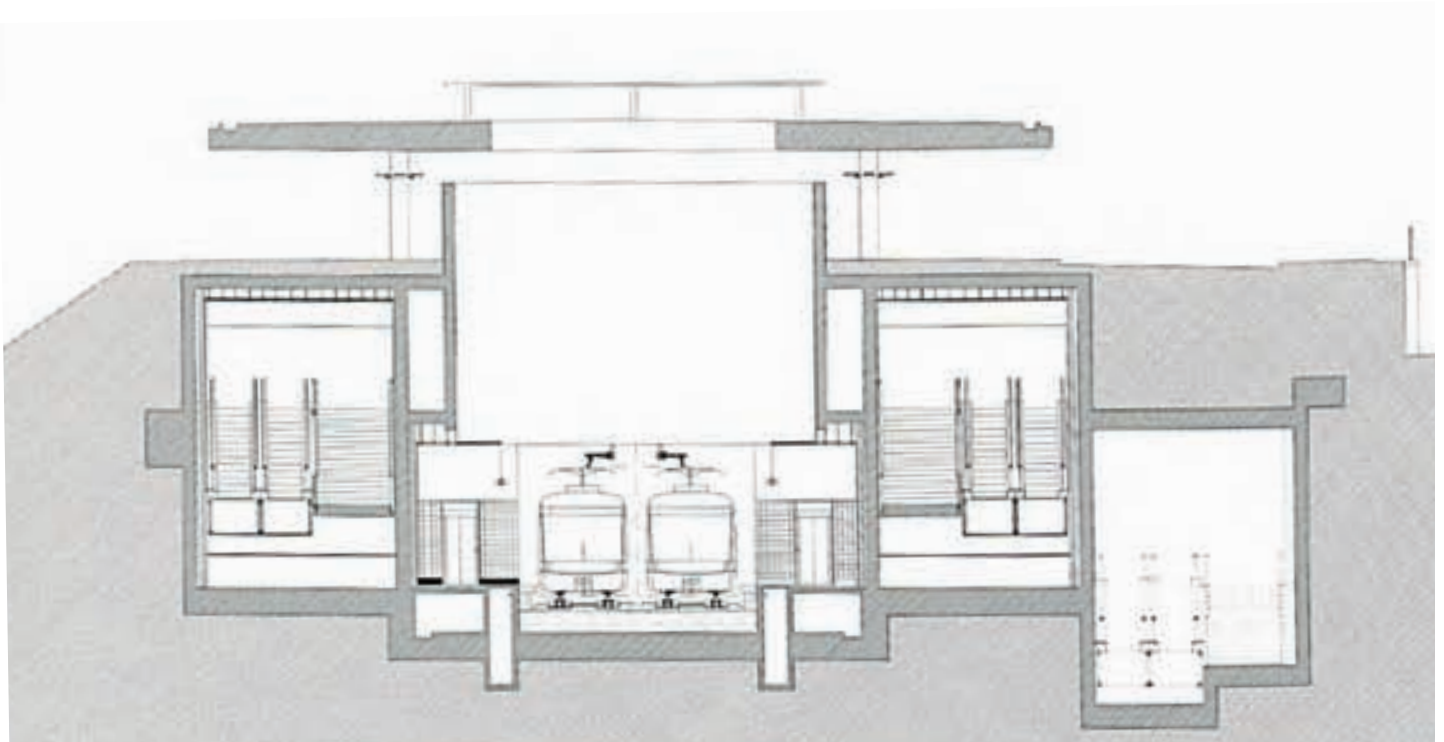
coupe transversale
