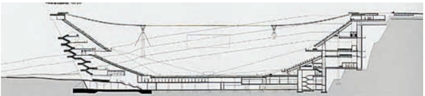
coupe transversale
