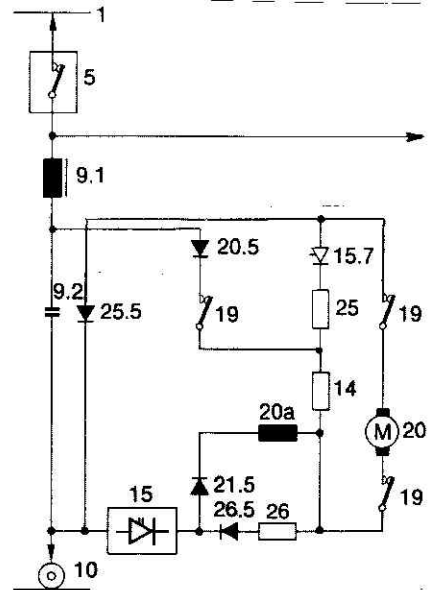
Montage BBC (freinage combiné)
